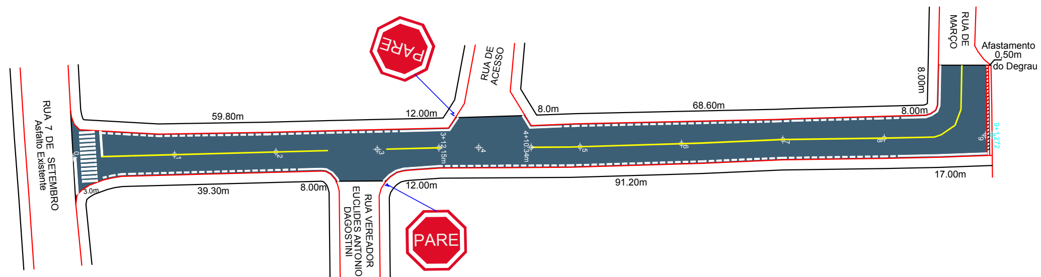
PLANTA SINALIZAÇÃO ESTACA O.P.P ATÉ 9+1.272m ESCALA: 1/750
